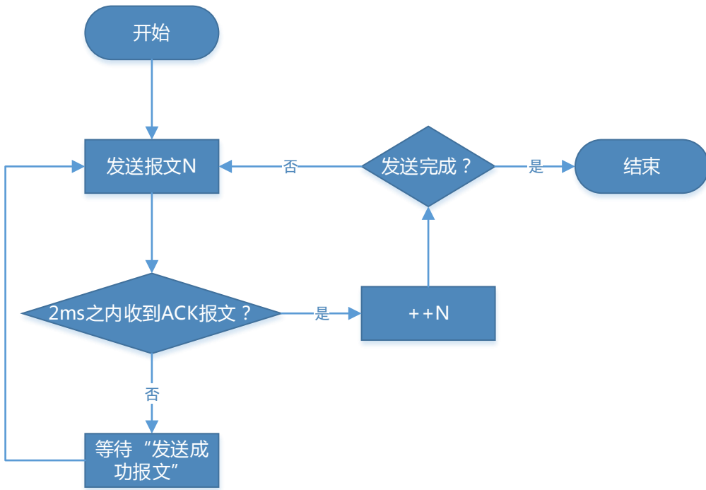
设置了ACK报文和“无线发送成功报文”的连续发送流程图
